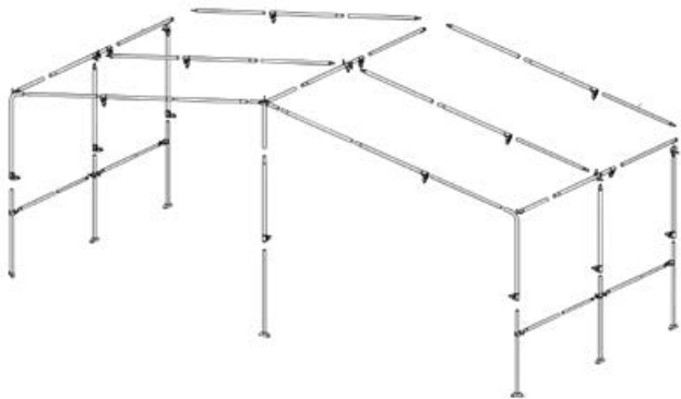
▲ Standaard frame uitvoering Parasol HD.
